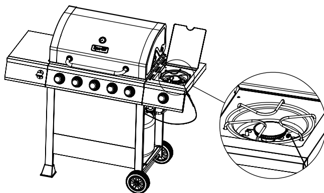
Quemador principal de cerillos/fósforos
