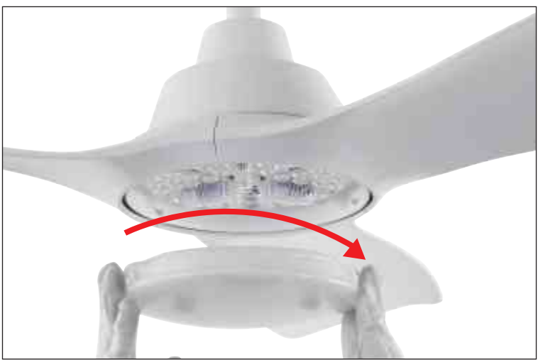
Paso 20 Gire la cubierta de la luz hasta que quede fija.
