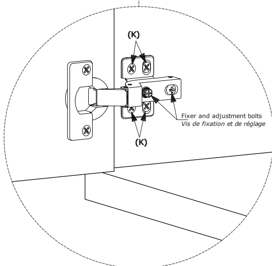
DETAIL 5 DÉTAIL 5
