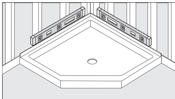
FIG 1 Vérifiez pour vous assurer que le bac est de niveau, en plaçant un niveau en position horizontale sur le dessus du seuil (bord avant) du bac, des côtés et de l'arrière.
