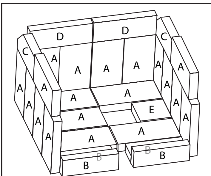
Figura 17 Patrón de montaje de ladrillos refractarios para estufa mediana
