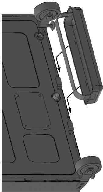
Right to left installation for models with wheels. Installation de droite à gauche pour les modèles à roulettes. Instalación de derecha a izquierda para modelos con ruedas.
