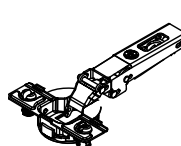
Bisagra de 105°
