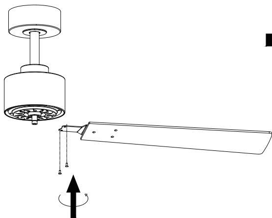
Installation fan blade diagram
