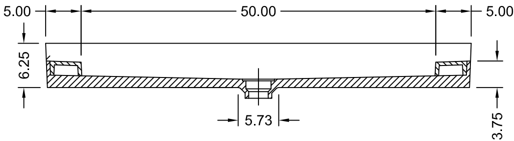
SECTION A-A
