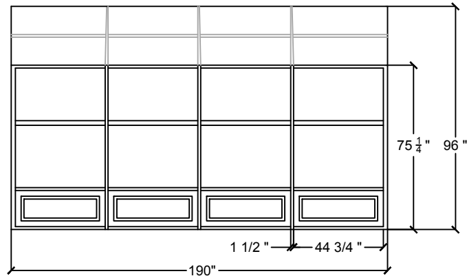
VUE DE CÔTÉ (LONGUEUR) SIDE VIEW (LENGTH)
