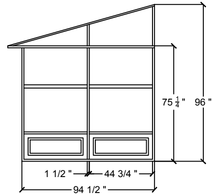
VUE DE CÔTÉ (LARGEUR) SIDE VIEW (WIDTH)
