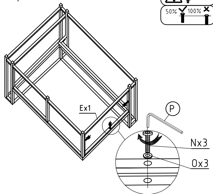
Step 9
