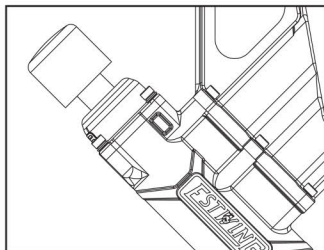
Tapa del martillo (Posición hacia arriba)
