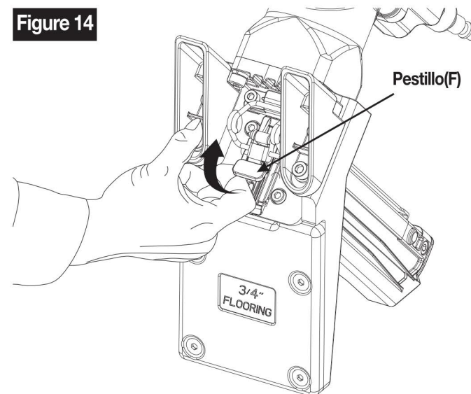
Tapa del martillo (Posición hacia abajo.)
