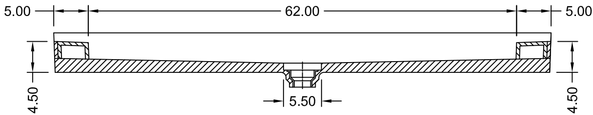
SECTION A-A
