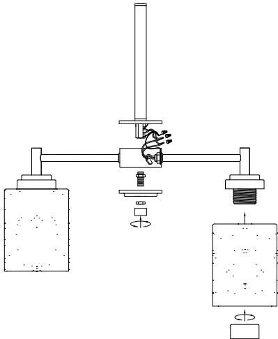
CONFIGURACIÓN DE DOWNLIGHT OPCIONAL OPTIONAL DOWNLIGHT SETUP
