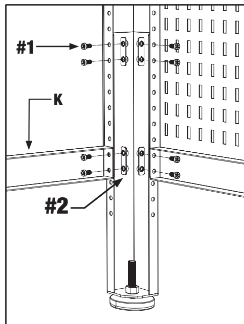
PATA TRASERA
