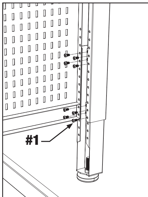
PATA DELANTERA
