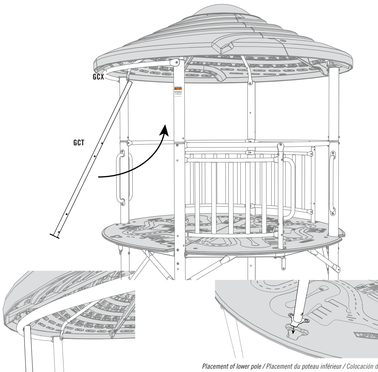
Placement of upper pole / Placement du poteau supérieur / Colocación del poste superior
