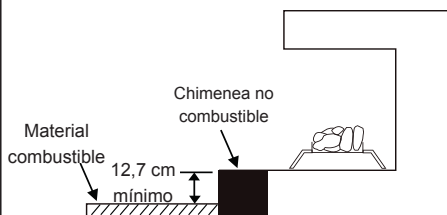
Fig. 9: Distancias de separación mínimas de la chimenea sobre los pisos combustibles
