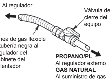
Fig. 16: Conexión de la línea de gas flexible a la válvula de cierre del equipo
