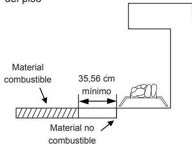
Fig. 8: Distancias de separación mínimas si la instalación es al nivel del piso
