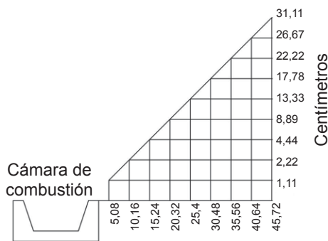
Fig. 4: Distancia mínima de separación del combustible a las paredes
