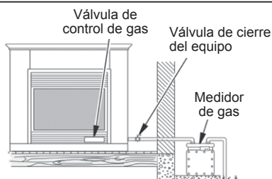
Fig. 18.2: Verificación de las juntas de gas (solo gas natural)
