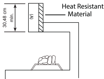
Fig. 5: Materiales resistentes al calor (azulejo de pizarra, mármol, baldosas, etc.) sobre la chimenea
