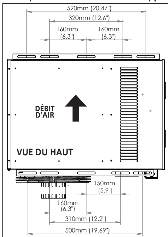
MHU50/MHU80 Dimensions du Support
