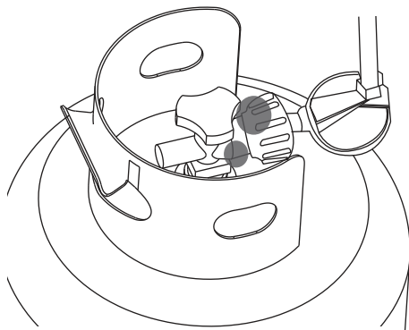
connexion bouteille - régulateur (figure 9)
