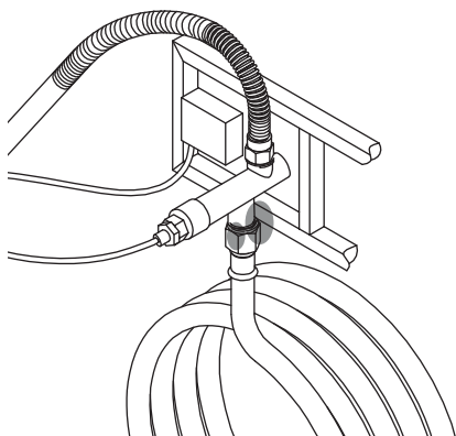
connexion vanne de gaz - tuyau (figure 11)
