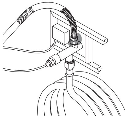
connexion vanne de gaz - soufflet (figure 10)
