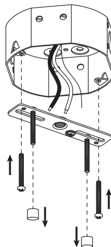
Wire Nuts
