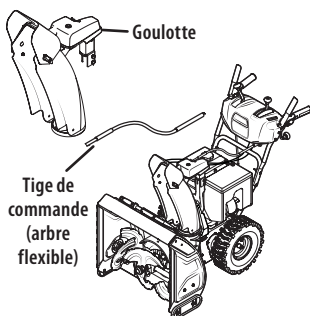
Commande supérieure avec arbre flexible, goulotte en acier et commande de déflecteur à 2 directions à la page 70
