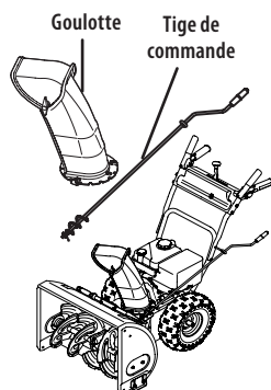
Commande latérale de rotation et commande manuelle de déflecteur à la page 67
