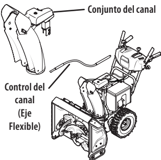
"Control del Canal Superior (Eje Flexible) c/ Canal de Acero y Control de Inclinación de 2 Direcciones" on page 40
