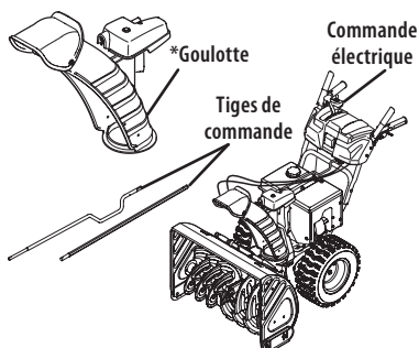
Commande supérieure électrique et commande de déflecteur à 4 directions à la page 72
