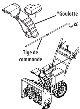
Commande supérieure de goulotte et commande manuelle de déflecteur à la page 68
