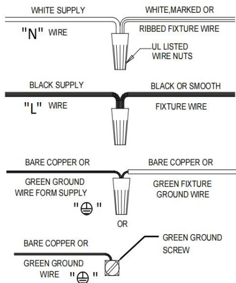
Step 2: Wiring
