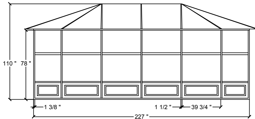
VUE DE CÔTÉ (LONGUEUR) SIDE VIEW (LENGTH)
