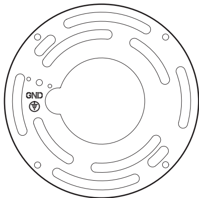
Placa de montaje (preinstalada, no está a escala)
