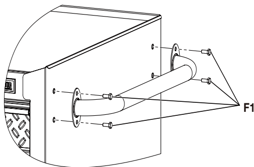
F1. Boulons à tête hexagonale (M6 - 1,00 x 15)
