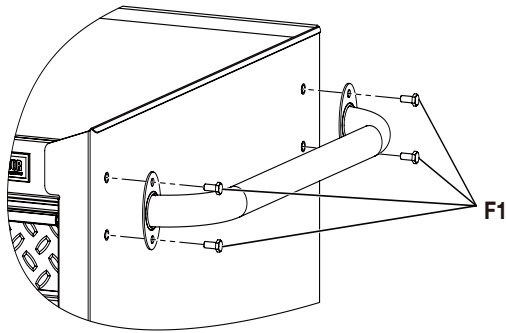
F1. M6 - 1.0 x 15 hex bolt
