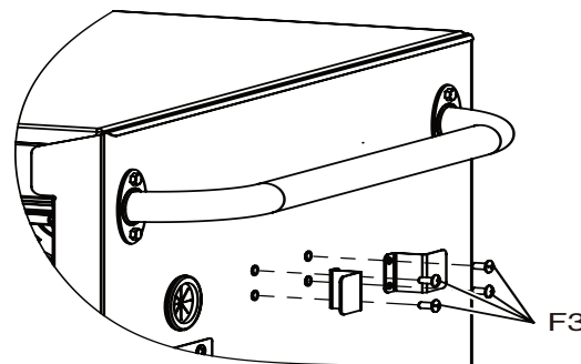
F3. Vis cruciforme (M6 - 1,00 x 12)
