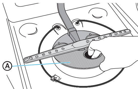
Ⓐ Filtre fin
