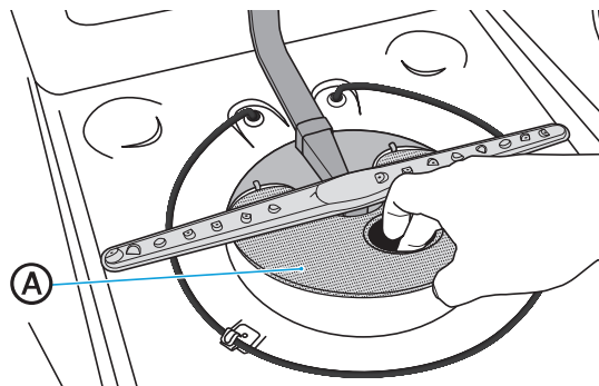
Ⓐ Filtro fino
