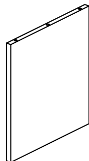
BOTTOM DIVIDER (L&R Same) QTY 3
