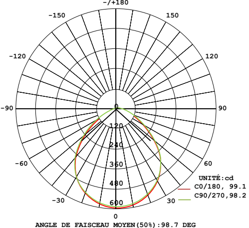
61433D DIAGRAMME
