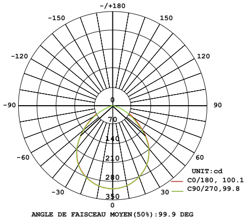
6733D DIAGRAMME
