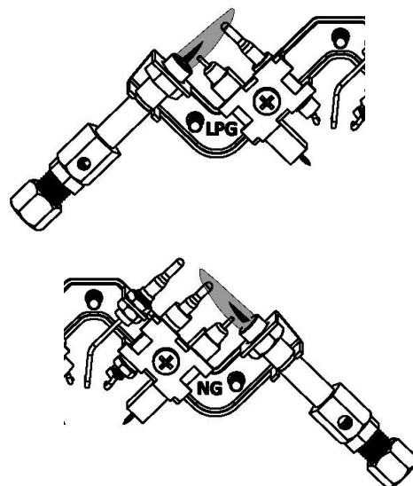
Fig. 21: Piloto
