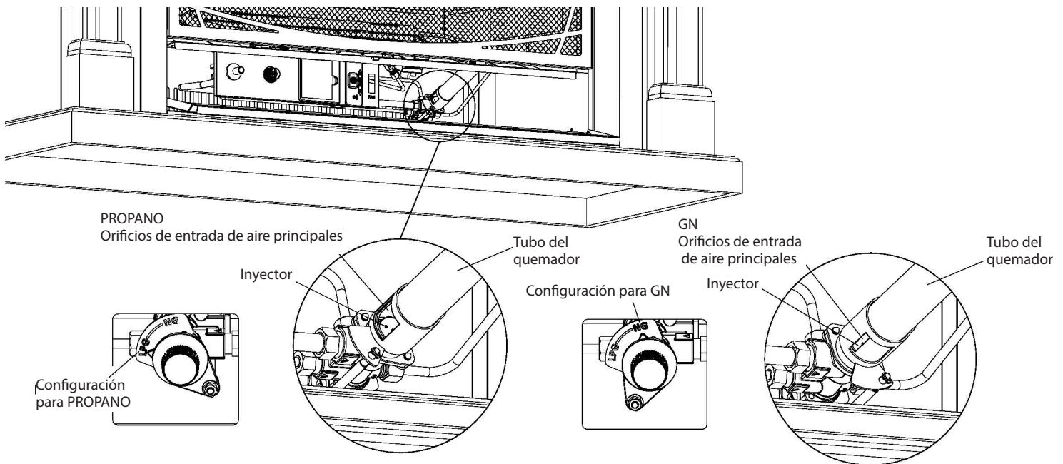
Fig. 36—Entrada de aire principal en el calentador
