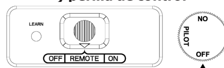
Fig. 20—Receptor y perilla de control
