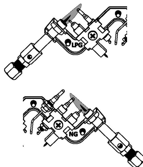
Fig. 21—Pilot
