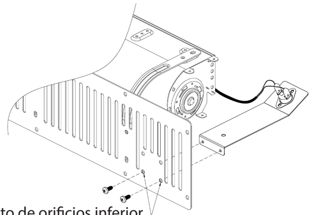
Fig. 7—Fijación del soporte del interruptor térmico
