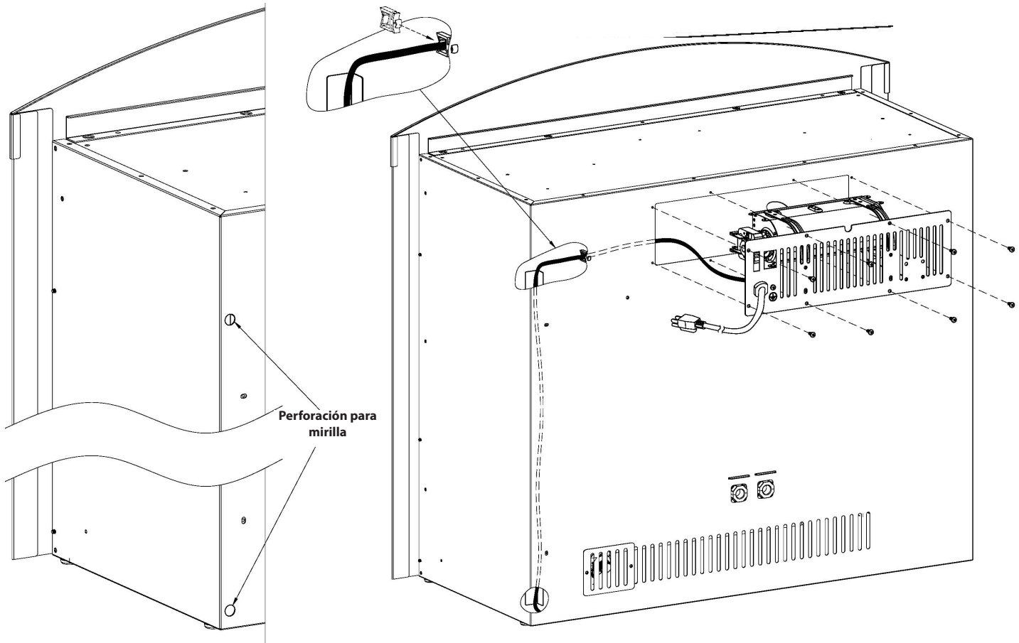
Fig. 8—Tendido de cables y accesorio del soplador
