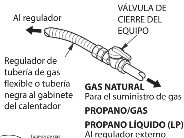
Fig. 16—Conexión de la línea de gas flexible
