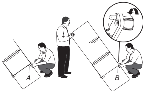
A. Ôter le dispositif de nivellement. B. Installer le dispositif de nivellement.
