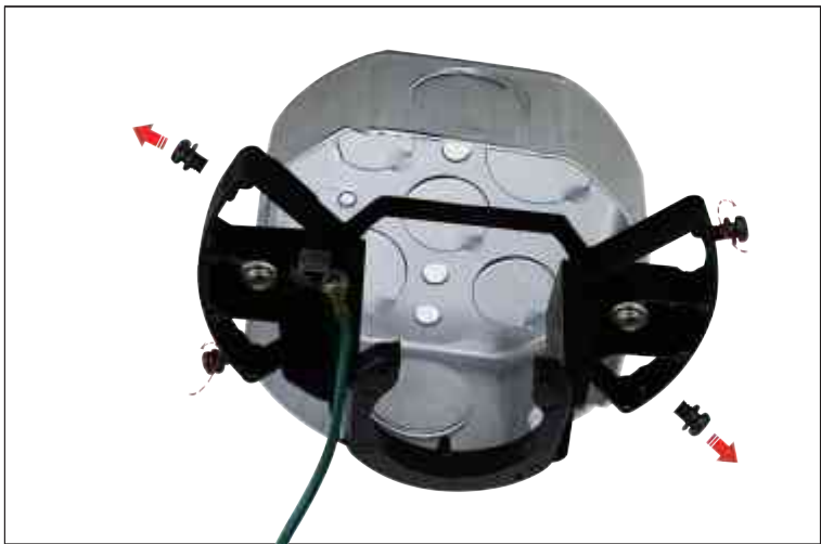
Paso 7 Retire 2 tornillos opuestos y loosn los otros 2 tornillos.
