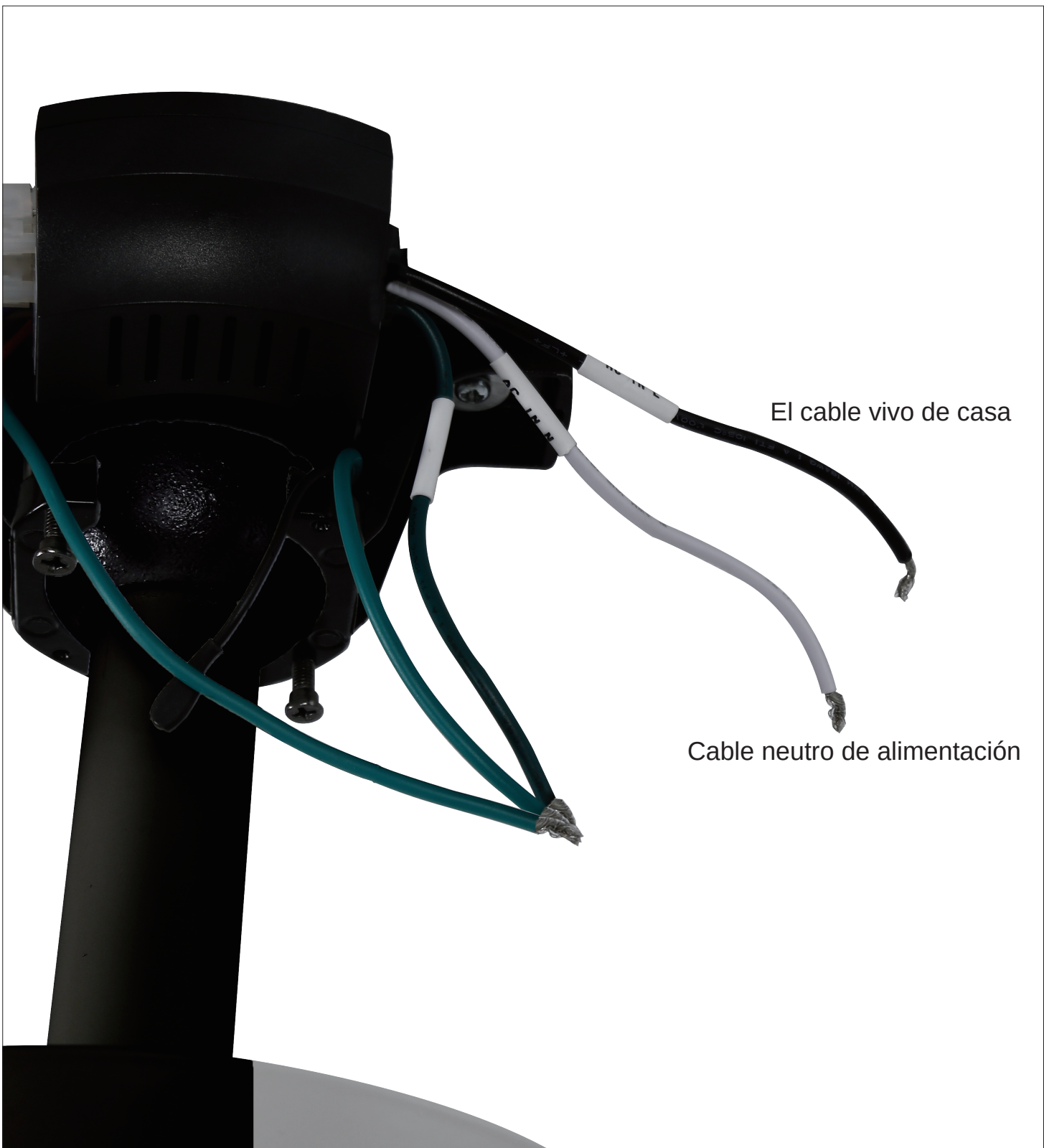
Paso 10 Conecte los cables del otro lado del receptor al circuito doméstico.
