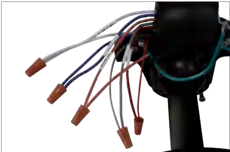
Psao 9 Conecte los cables del mismo color del el ventilador y el receptor.
