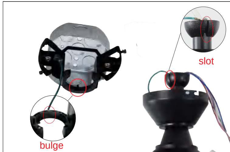
Paso 8 Cuelgue el ventilador en el soporte de suspensión y alinee la ranura de la varilla inferior con la protuberancia del soporte de suspensión.
