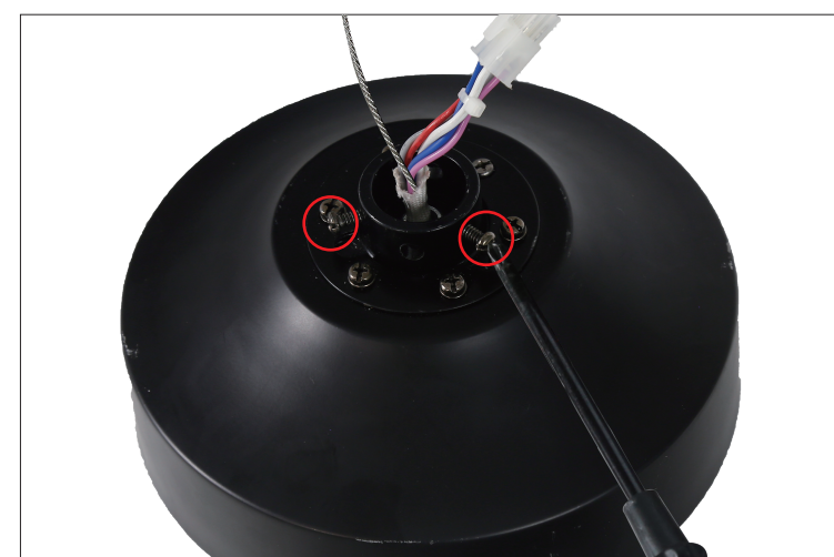
Paso 2 Afloja los dos tornillos del acoplador.
