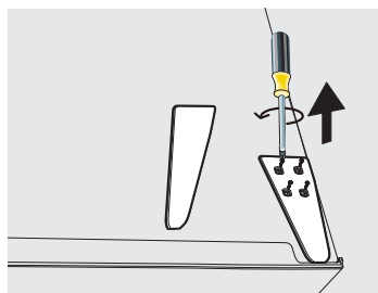
Retirez la charnière supérieure droite
