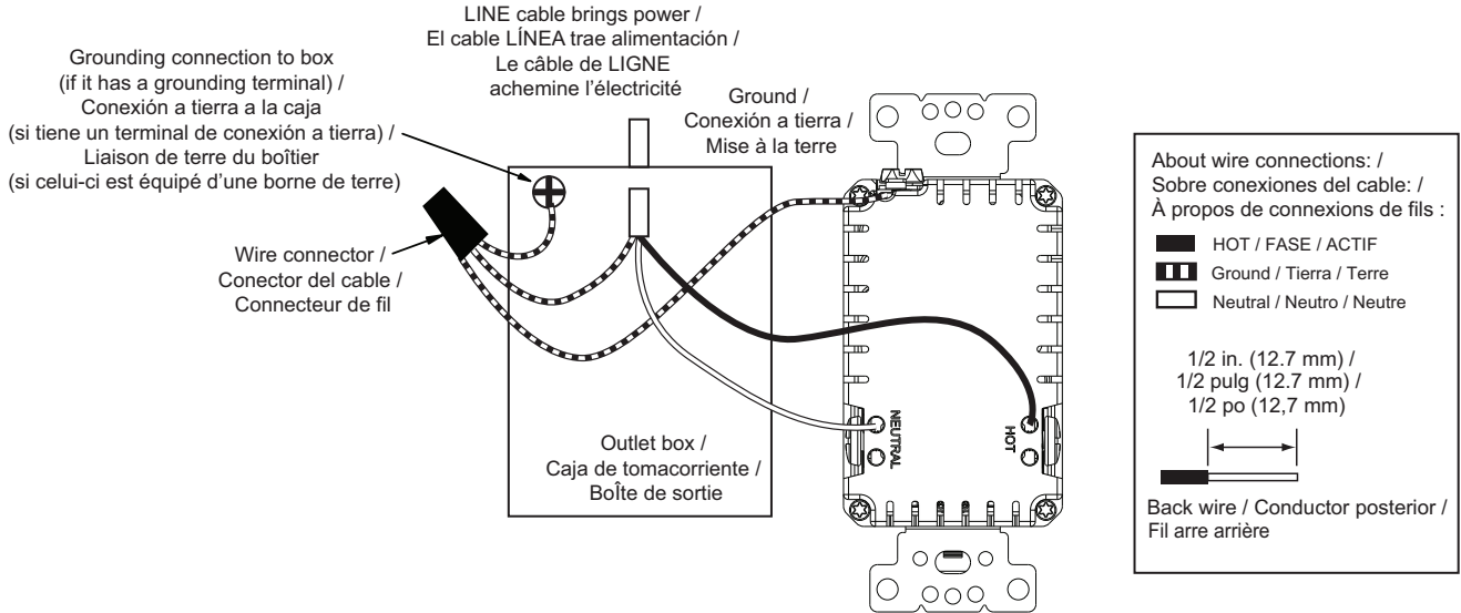
Figure / Figura / Figure 1 : Wiring Diagram / Diagrama de alambrado / Schéma de câblage
