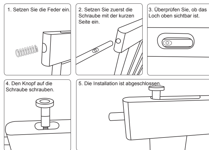
180° Schwingtür
