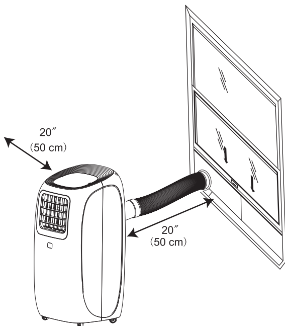
Instalación en ventana corrediza vertical
