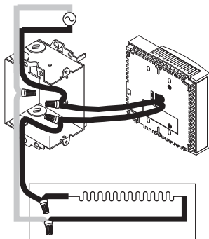
Instalación de 4 cables
