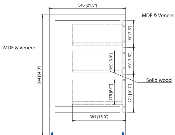
Side / Côté
