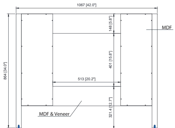
Back / Derrière
