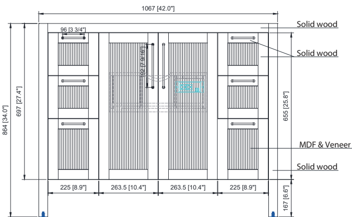
Front / Devant
