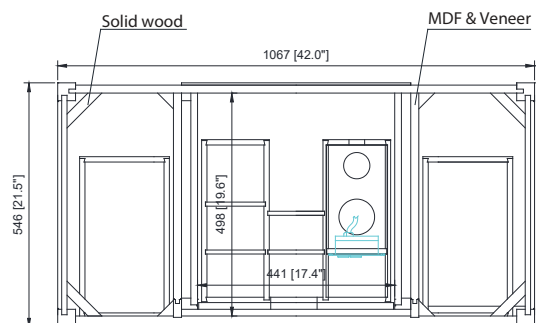
Top / Haut
