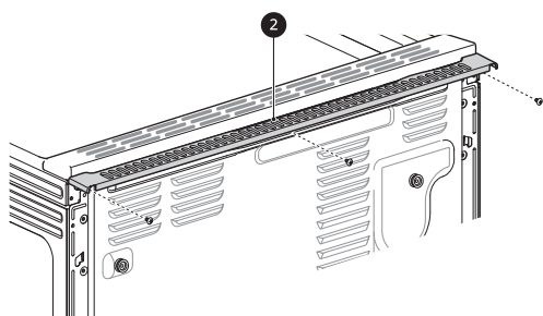
2 Placa trasera
