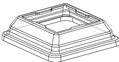
G2 | POST FOOT - A4M01279 (4) | 2 5/8"x9 7/8"x9 7/8" (68x250x250)
