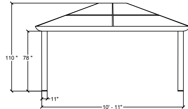
VUE DE CÔTÉ (LARGEUR) SIDE VIEW (WIDTH)
