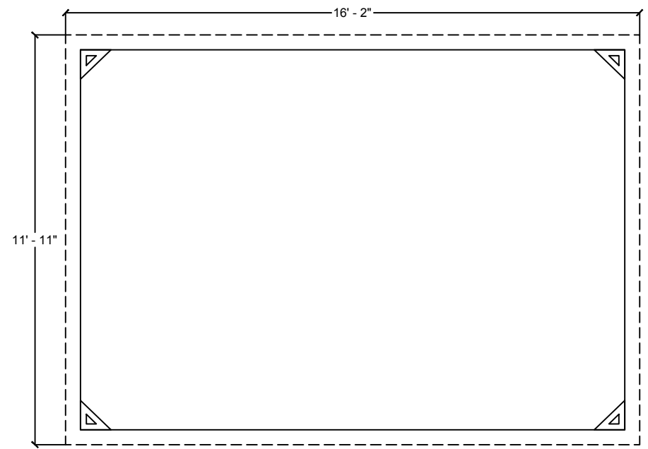
REBORD DU TOIT ROOF OVERHANG
