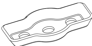
Mounting Bracket Support de fixation Abrazadera de montaje
