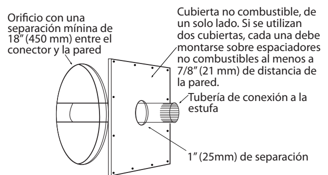
Figura 7: SOLO PASADOR DE PARED APROBADO PARA CANADÁ
