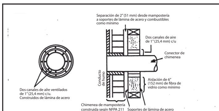
Figura 11 (EE. UU. SOLAMENTE)
