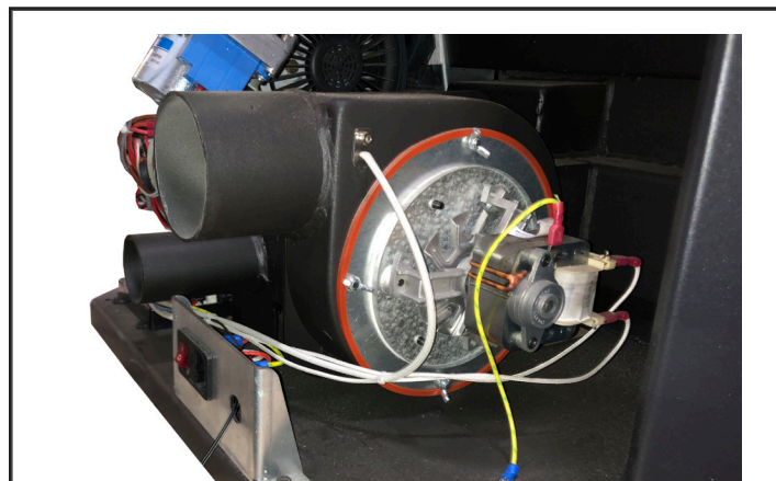
Figura 26: Soplador de escape de H3W80XL
