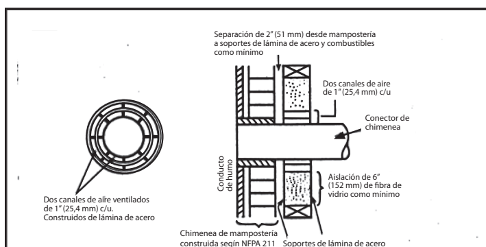
Figura 10 (EE. UU. SOLAMENTE)
