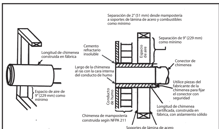
Figura 9 (EE. UU. SOLAMENTE)
