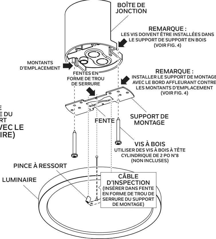
Fig. 3 INSTALLATION SUR LA BOÎTE DE JONCTION DU VENTILATEUR DE PLAFOND EN FORME DE L
