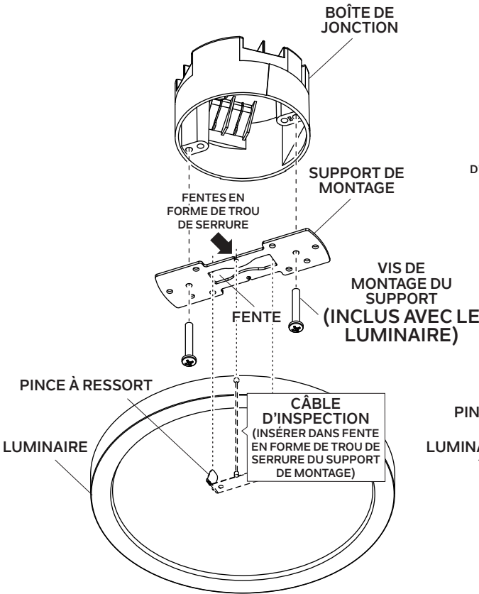
Fig. 2 INSTALLATION SUR LA BOÎTE DE JONCTION DU VENTILATEUR DE PLAFOND RONDE
