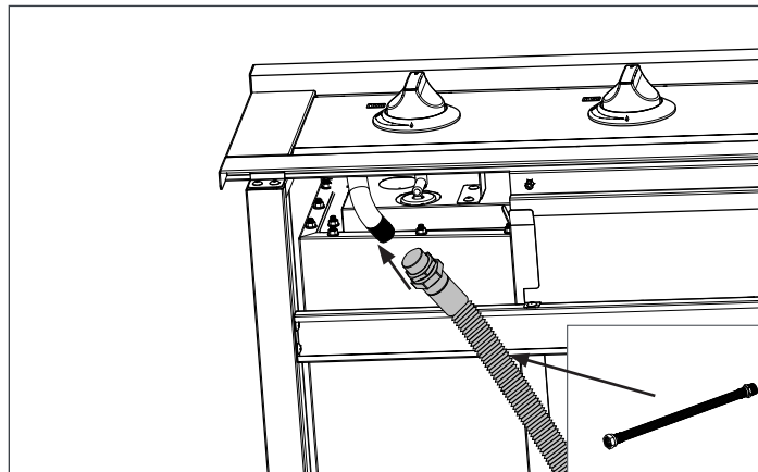
Tuyau d'extension ondulé en métal
