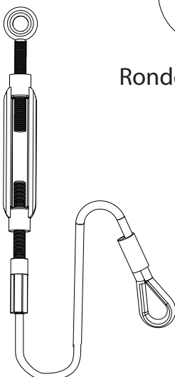
Assemblage de câble avec tendeur - 4 pieds
