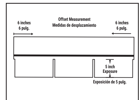
Fig. 5 Offset Measurement Medidas de desplazamiento
