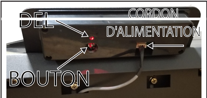
Figure 16 Dos de l'afficheur
