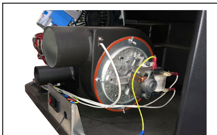
Figure 27 Ventilateur d'échappement du modèle PSBF66W
