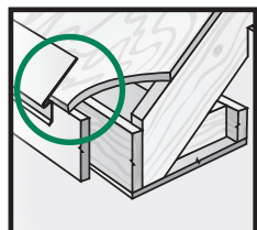
Figure 10 Drip Edge
