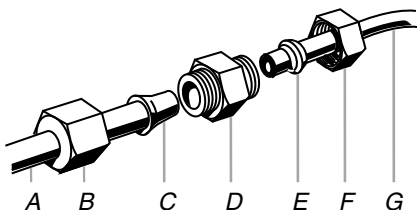
A. Tubería de agua del refrigerador B. Tuerca (provista) C. Bulbo D. Acoplamiento (adquirido) E. Féula (adquirida) F. Tuerca (adquirida) G. Línea de agua de la casa
