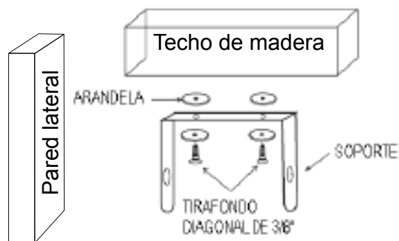
Figura 4b. Montaje de dos tornillos
